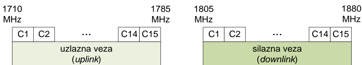
Slika 1 - Grafički prikaz raspodjele radio-frekvencija iz opsega 1710-1785/1805-1880 MHz za GSM/DCS1800 i MFCN sisteme
