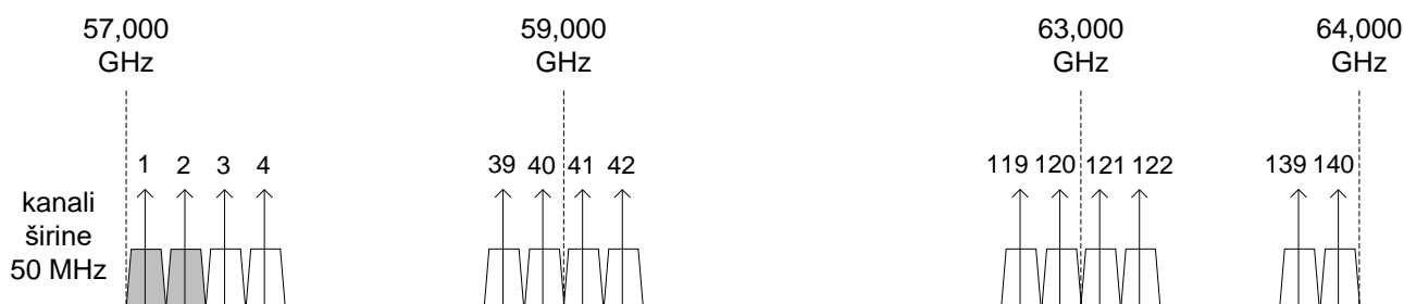
Slika 1 - Grafički prikaz kanalnog aranžmana u opsegu 57-64 GHz za fiksne veze
